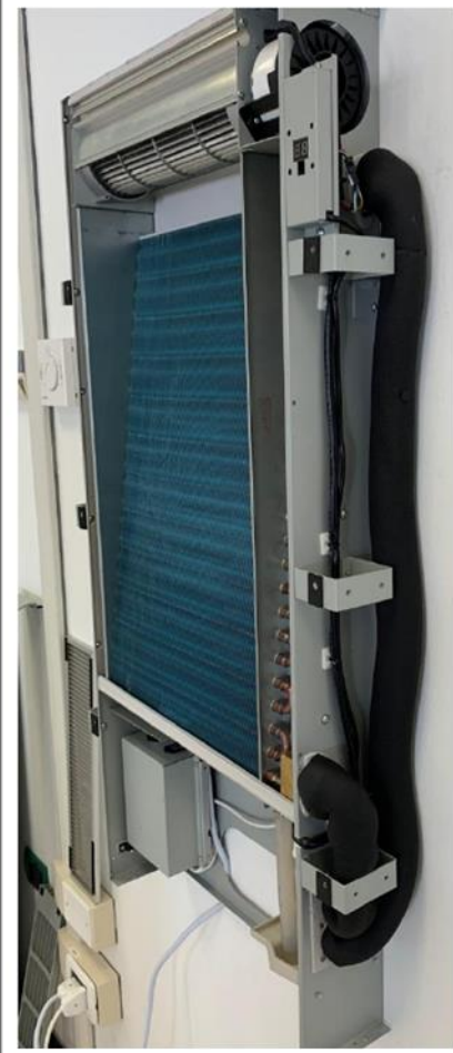
POSIZIONARE ISOLAMENTO ESTERNO DELLE TUBAZIONI
